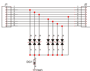
Fig1.-Esquema eléctrico / Electrical diagram
