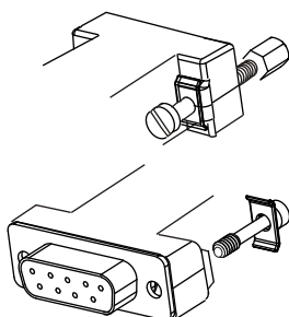
Fig2. Disposición de tornillería suministrada con el protector / Disposition of the screws provided with the protector.
