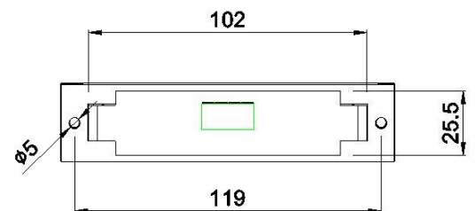
開孔尺寸
